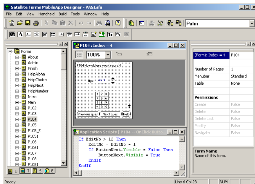
รูปที่ 6 ตัวอย่างการพัฒนาโปรแกรมบนปาล์มโดยใช้ Satellite Forms
